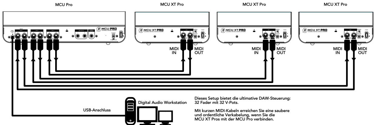
Verkabelung 1: USB
