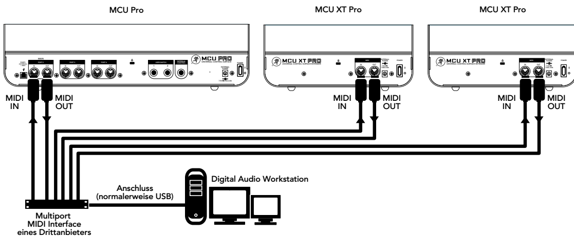
Verkabelung 2: MIDI
