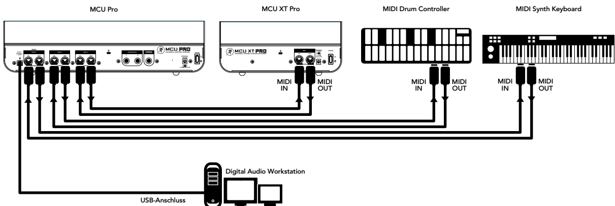
Verkabelung 3: mit mehreren MIDI-Geräten
